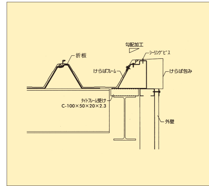
■ 妻側(ケラバ)納め図
