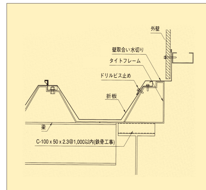
■ 壁取合い納め図
