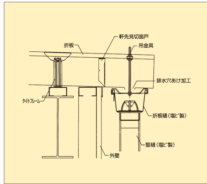
■ 軒先・雨樋納め図 (単位: mm)
